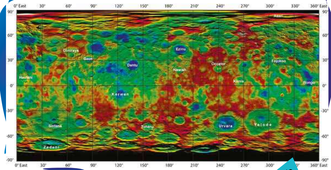
Мал. 9. Мапа Церери
